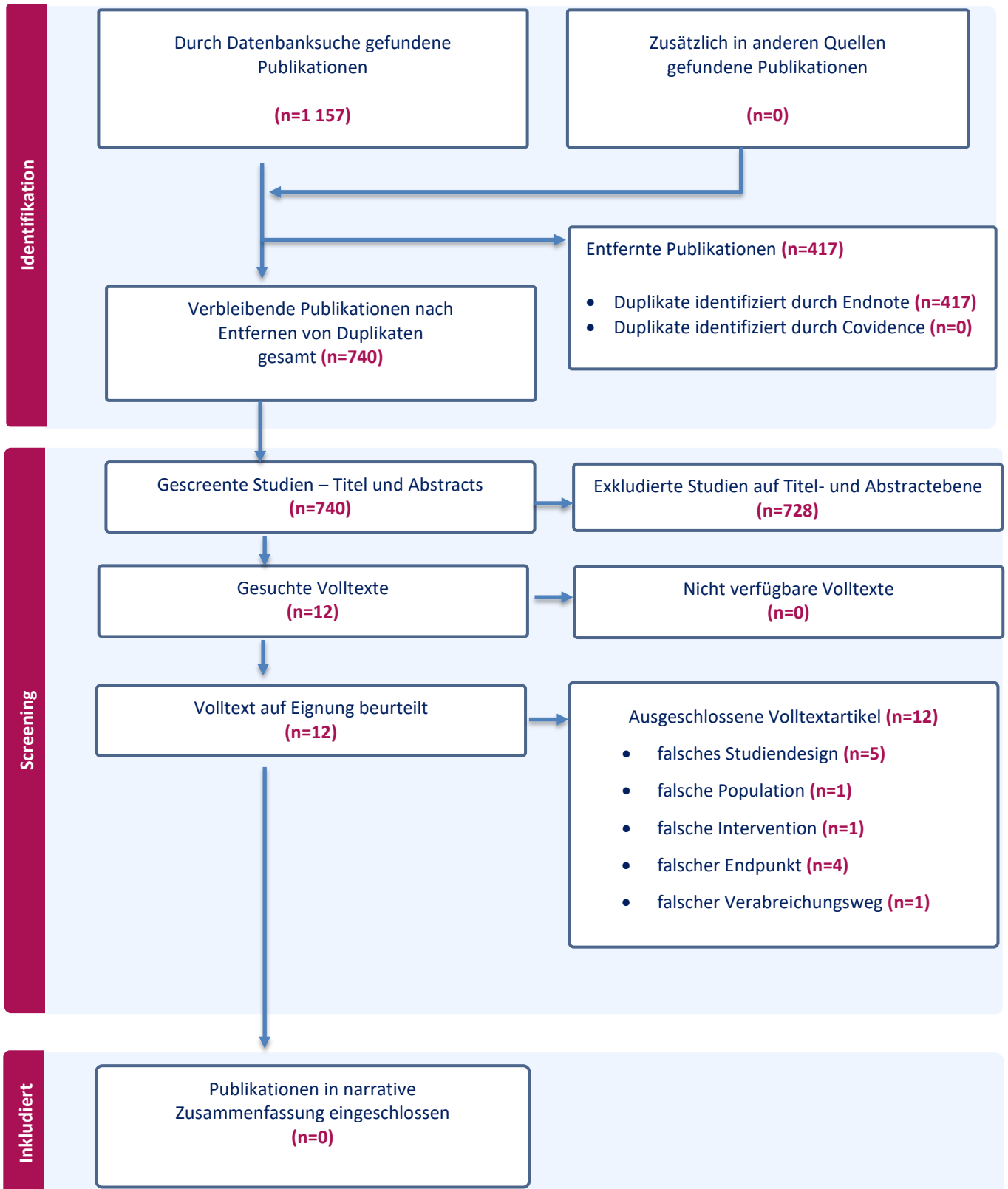
Abbildung 1: PRISMA-Flussdiagramm modifiziert (10)
